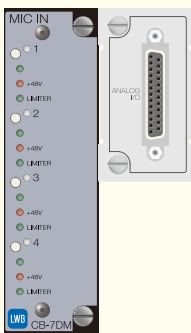
CB-7DM マイク入力モジュール (D-sub25)
