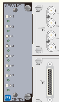
CB-7DY AES3 入出力モジュール (D-sub25/BNC)
