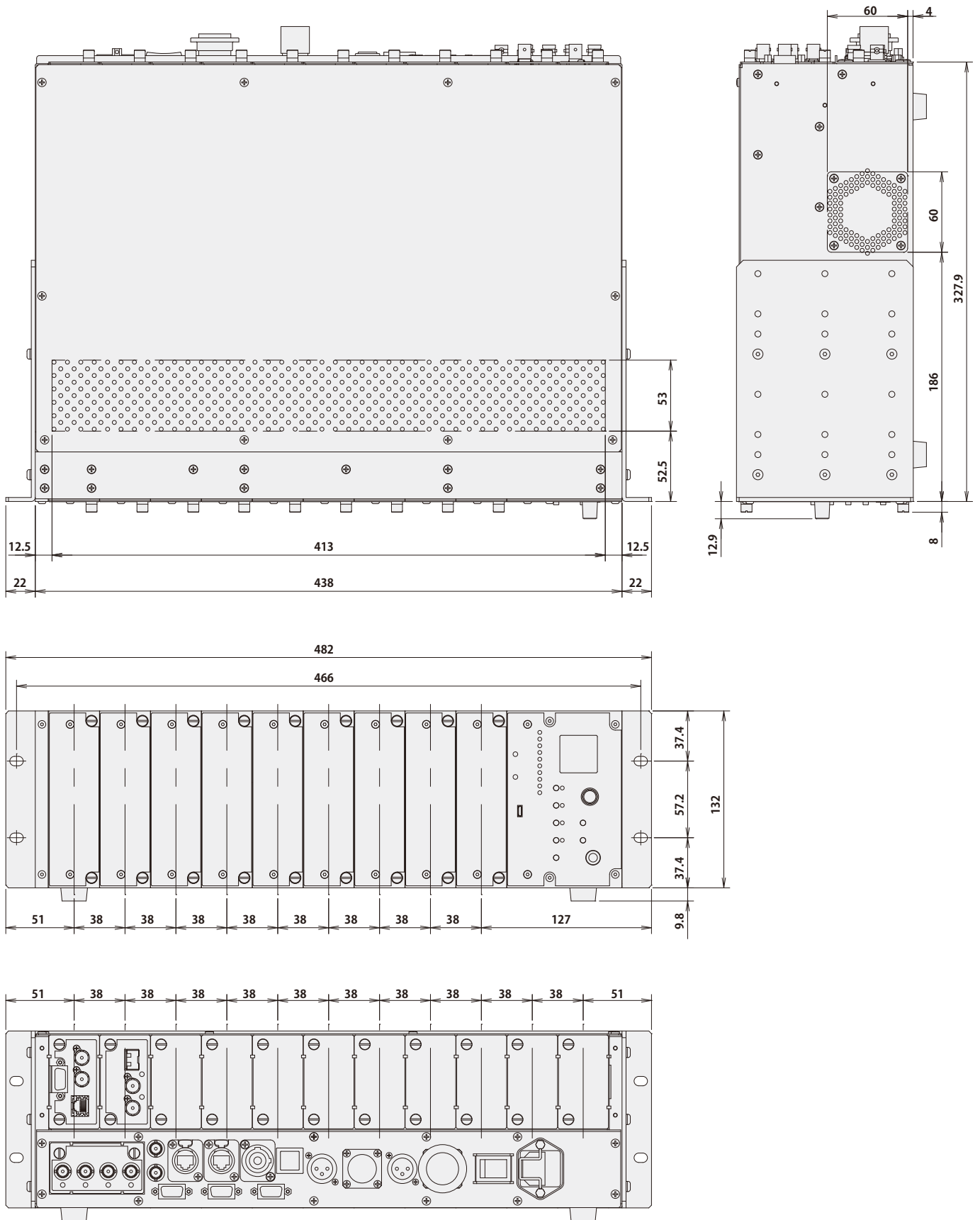
LWB-72 寸法図 (単位 : mm)
