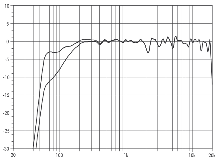
Y7P 周波数特性 標準、CUT 設定
