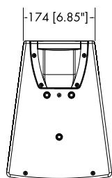
Y7P/Y10P キャビネット寸法 mm [インチ]
