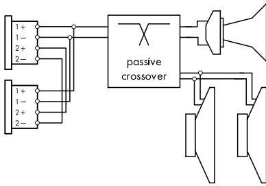
コネクターの接続
