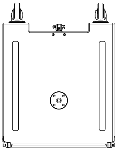
XSL-SUB キャビネット寸法 mm [インチ]* *同じ寸法が XSL-GSUB にも適用されます。
