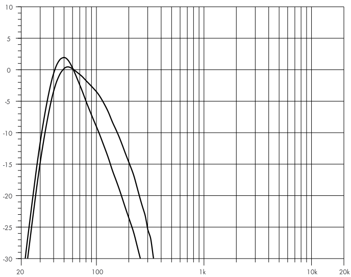
XSL-SUB 周波数特性 標準、INFRA モード
