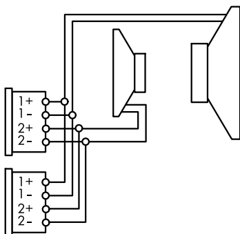
NLT4 F/M コネクターの結線
