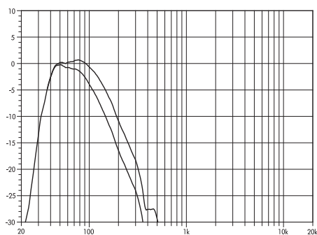
図 3: E15X 周波数特性、標準および 100 Hz 設定
