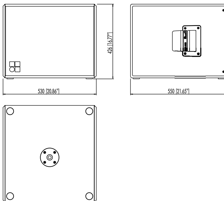
図 4: E15X-SUB キャビネットの寸法: 単位 mm (インチ)
