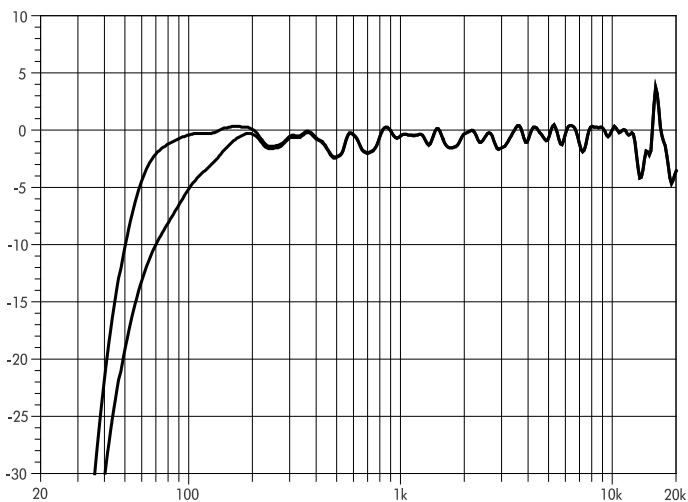
図 18: 10A-D 周波数特性 標準、CUT 設定
