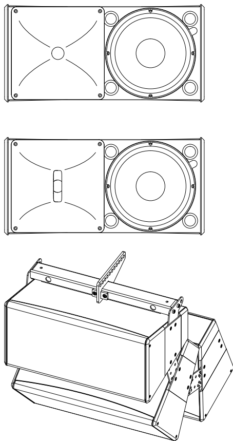
図 1: 10A/10A-D ラウドスピーカー リギング例:
