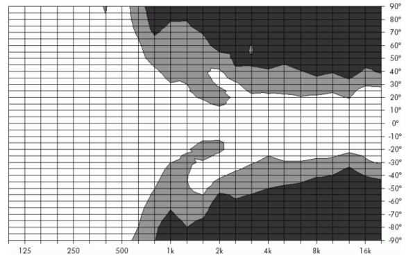
図 9: アイソバー、垂直
