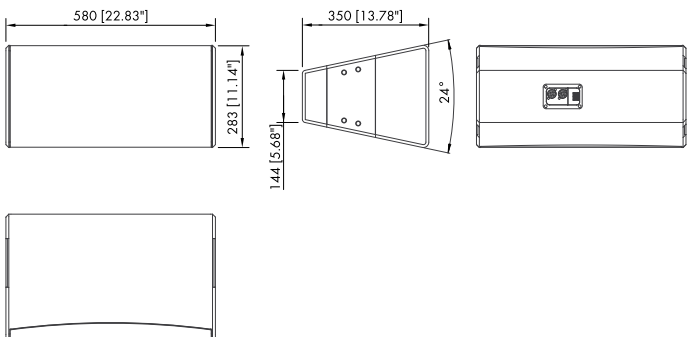
図 19: 10A/10A-D キャビネット寸法 mm [インチ]
